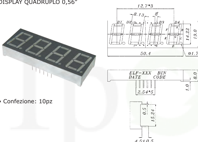
DISPLAY QUADRUPLA 0,56"
