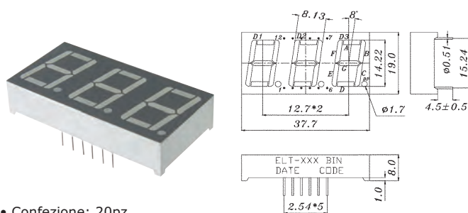
DISPLAY TRIPOLO 0,56"
